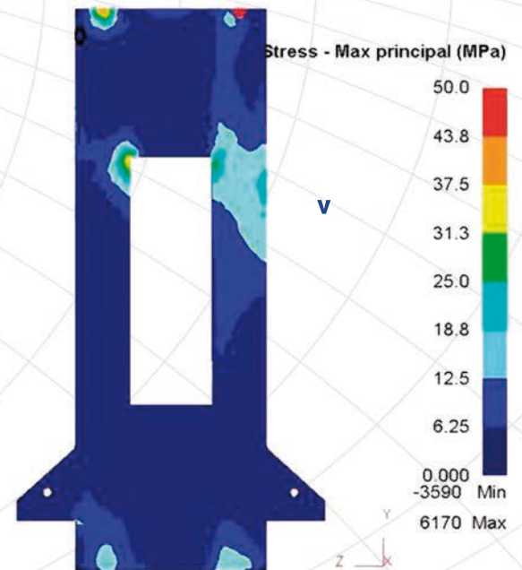
Análisis estructural de prensa y componentes
