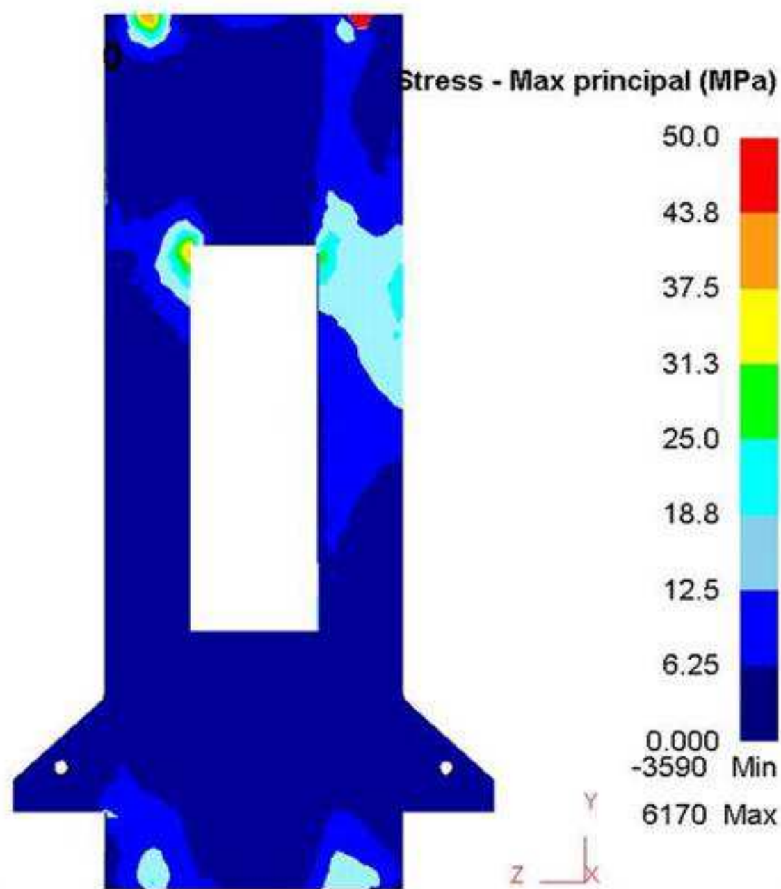
Análisis estructural de prensa y componentes.
